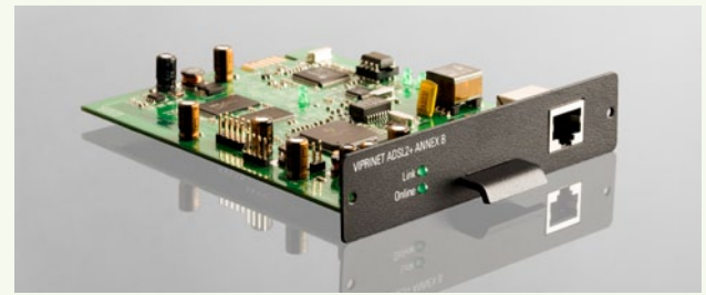
Bis zu 6 integrierte Leitungsmo-dems, die sich im laufenden Betrieb wechseln lassen
